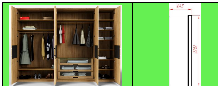
Габаритная глубина и высота шкафа
